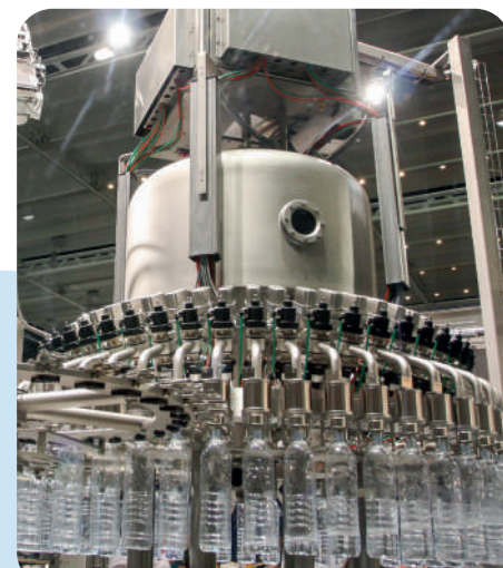
Embouteillage, sertissage.
